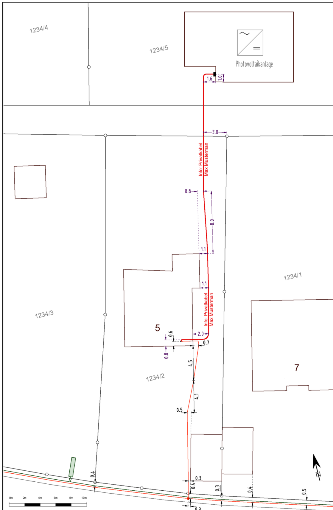
Beispiel aus unserem Geoinformationssystem (Privatleitung Strom für eine Photovoltaikanlage)
