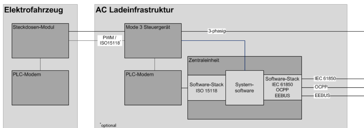
Abbildung 11: Schnittstellen Ladekommunikation
